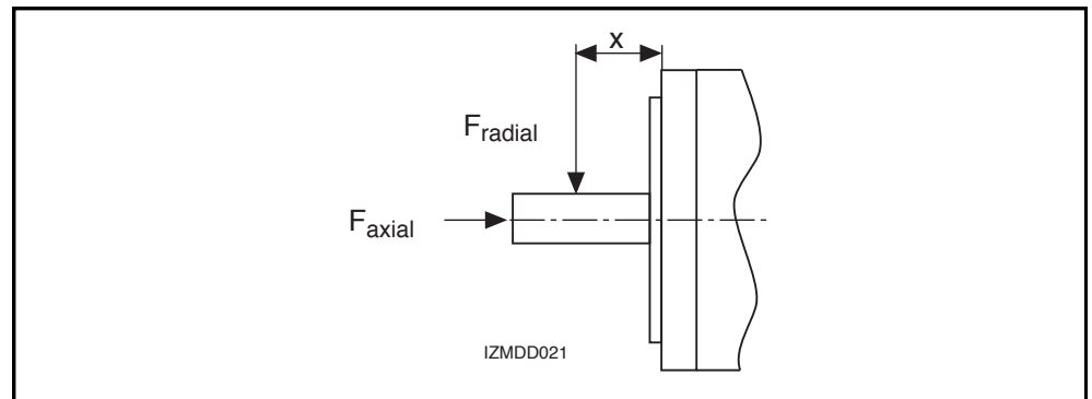
Fig 7.10: Shaft load
